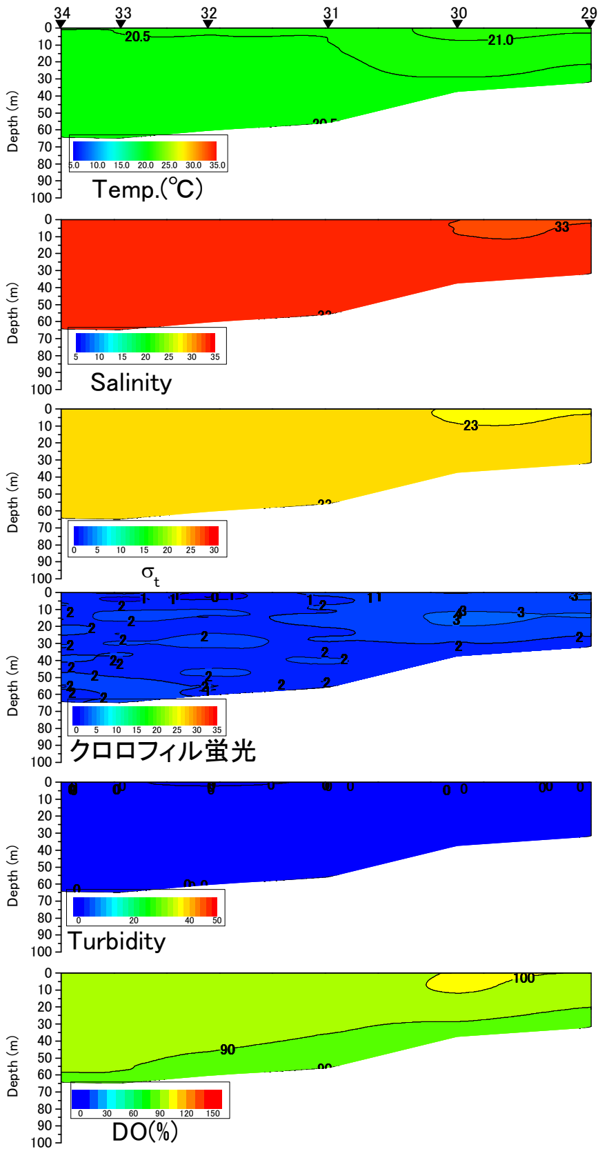
八代海西ラインの水温(°C)、塩分、密度( \sigma_t )、クロロフィル蛍光強度、濁度、溶存酸素飽和度(DO%)の鉛直面図(国土交通省の調査による) (2016年6月8日)
